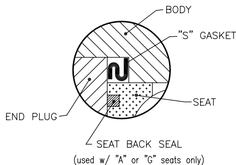
View A-A
