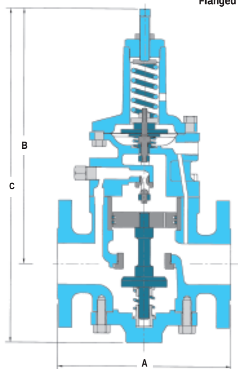
402/403 Flanged
